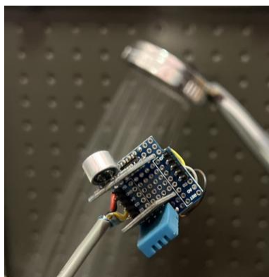
รูปที่ 8 ชุดเซนเซอร์วัด จากตำแหน่งที่ 3 ฝักบัว
