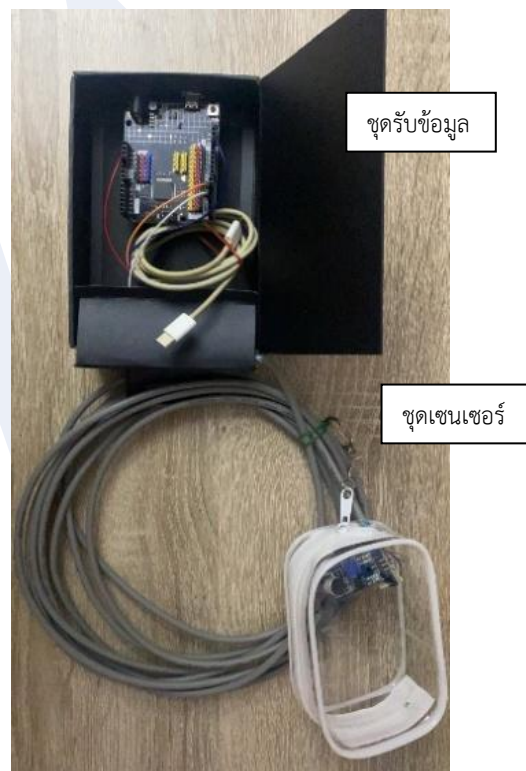
รูปที่ 5 ชุดต้นแบบระบบแจ้งเตือนความชื้นอุณหภูมิด้วยบอร์ด Arduino R4
