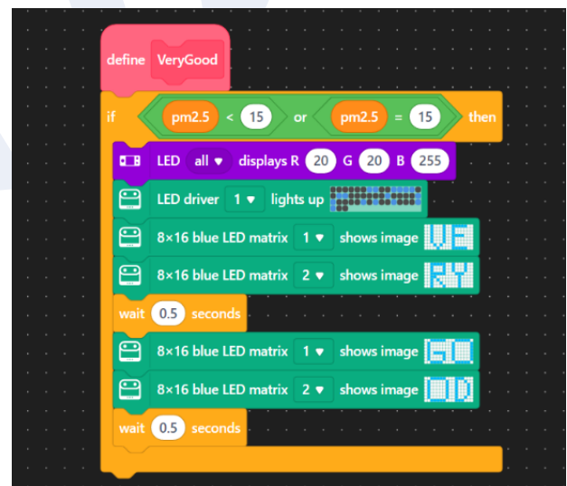
รูปที่ 5 ตัวอย่างชุดคำสั่งจากโปรแกรม mBlock
