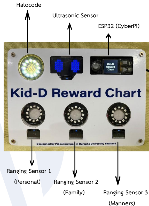
รูปที่ 1 ระบบการบันทึกคะแนนความดีดิจิทัลโดยใช้ IoT
