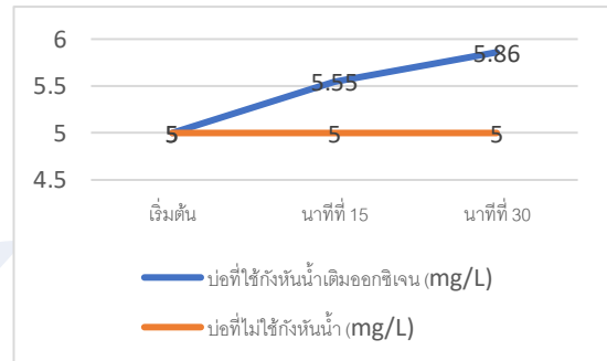
รูปที่ 7 กราฟเปรียบเทียบปริมาณออกซิเจนที่ละลายในน้ำ
