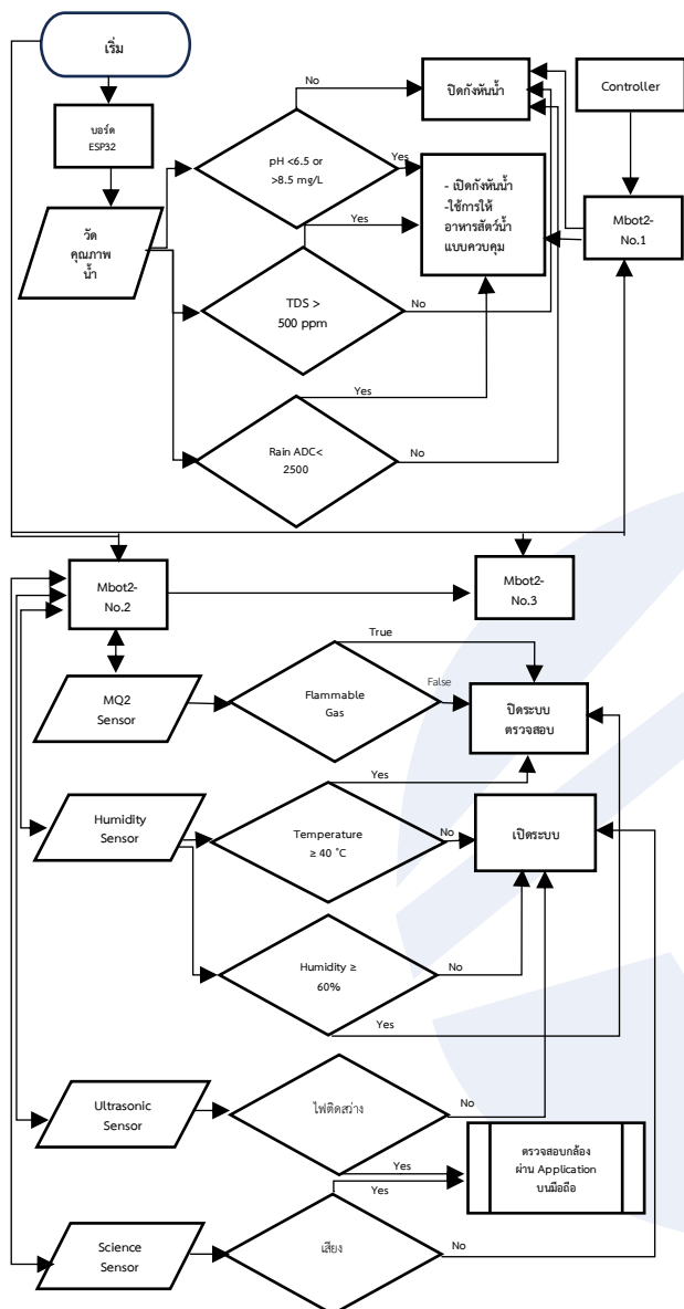
รูปที่ 4 แผนผังการทำงานของระบบเฝ้าระวังระบบนิเวศ ของบ่อน้ำสาธารณะ
