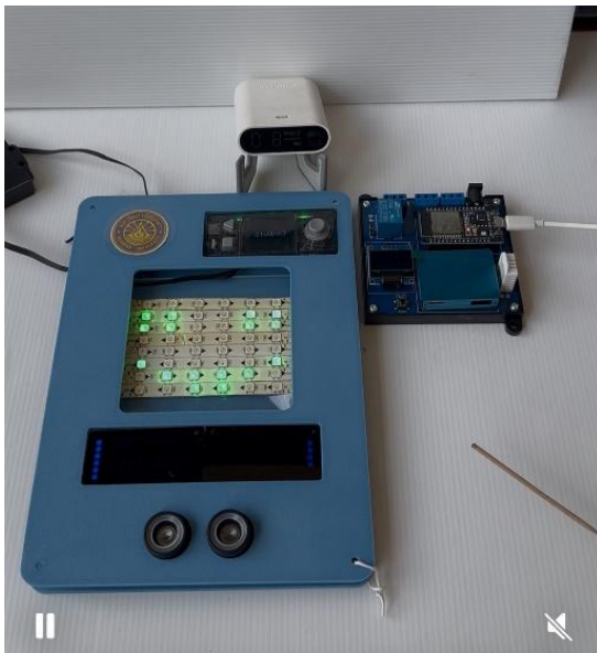
รูปที่ 6 แสดงการทดลองวัดค่าฝุ่น PM2.5 และการแจ้งเตือนอัตโนมัติโดยใช้ CyberPi
