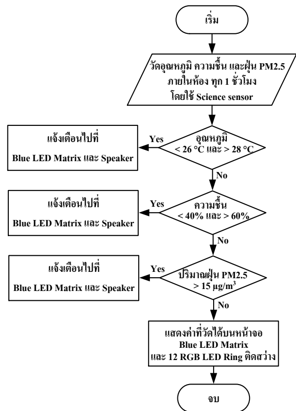
รูปที่ 5 แผนผังการทำงานของระบบแจ้งเตือนสภาพอากาศภายในห้องของเด็กเล็ก
