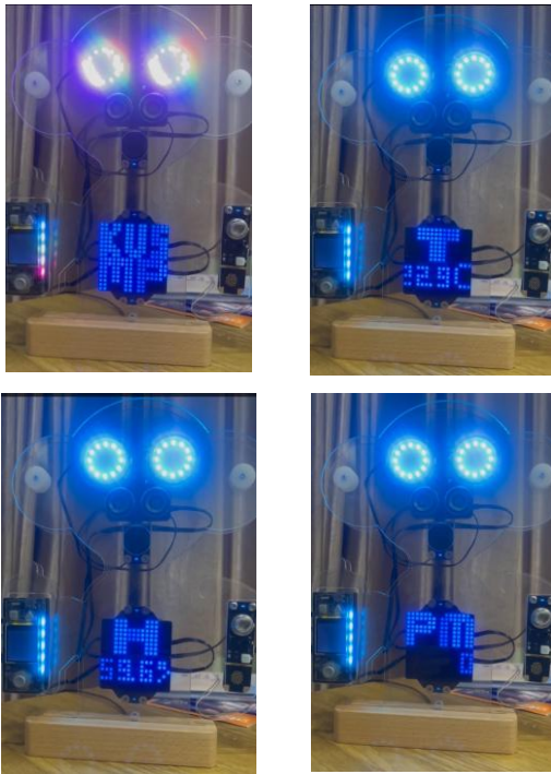
รูปที่ 6 ตัวอย่างการแสดงผลระบบแจ้งเตือนสภาพอากาศภายในห้องของเด็กเล็ก
