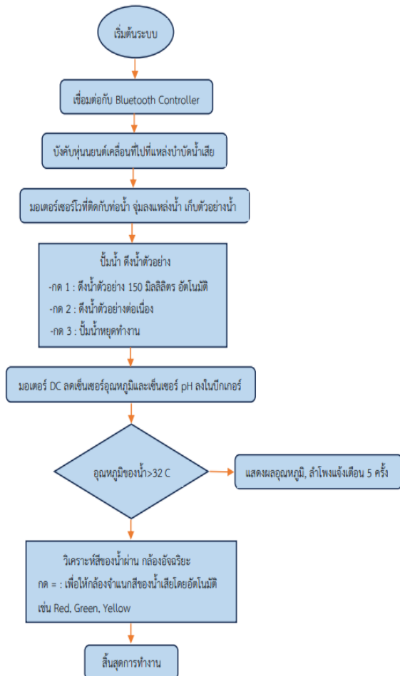
รูปที่ 5 Mbot2 (ควบคุมหุ่นยนต์และเก็บตัวอย่างน้ำ)
