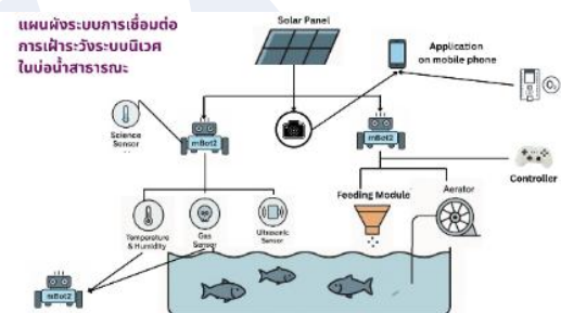
รูปที่ 3 แผนผังระบบการเชื่อมต่อระบบเฝ้าระวังระบบนิเวศของบ่อน้ำสาธารณะ
