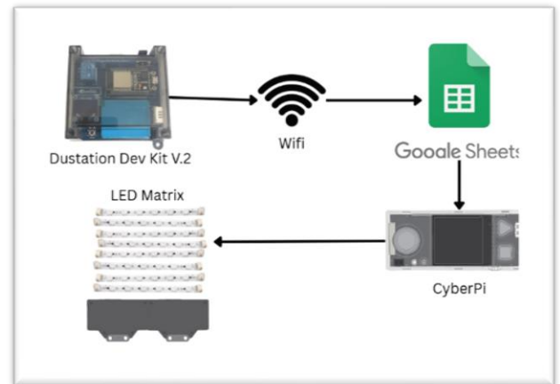
รูปที่ 4 แสดงส่วนประกอบและผังการเชื่อมต่อ
