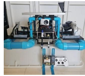
รูปที่ 2 การเชื่อมต่อระหว่างบอร์ด ESP32 และ Mbot 2 กับโมดูลเซ็นเซอร์ต่าง ๆ พร้อมกล้อง แสงโซล่าเซลล์ และรีโมทคอนโทรลเลอร์
