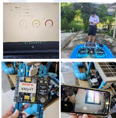
รูปที่ 5 การทดสอบระบบการทำงานของการเฝ้าระวัง ระบบนิเวศในบ่อน้ำสาธารณะ
