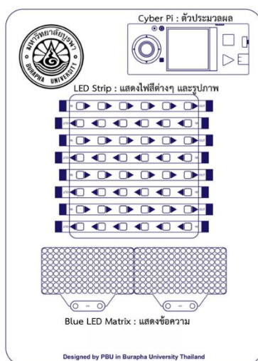
รูปที่ 3 แสดงส่วนประกอบภายในเครื่องแจ้งเตือนค่าฝุ่น PM2.5 อัตโนมัติ
