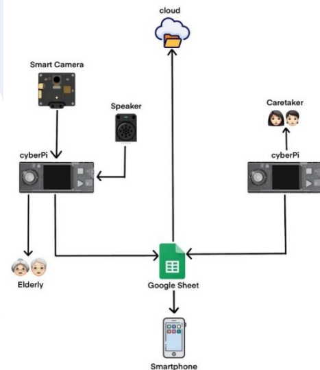
รูปที่ 4 แผนผังการเชื่อมต่ออุปกรณ์
